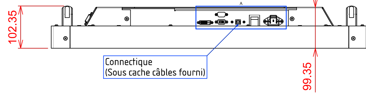
VUE DE DESSOUS
