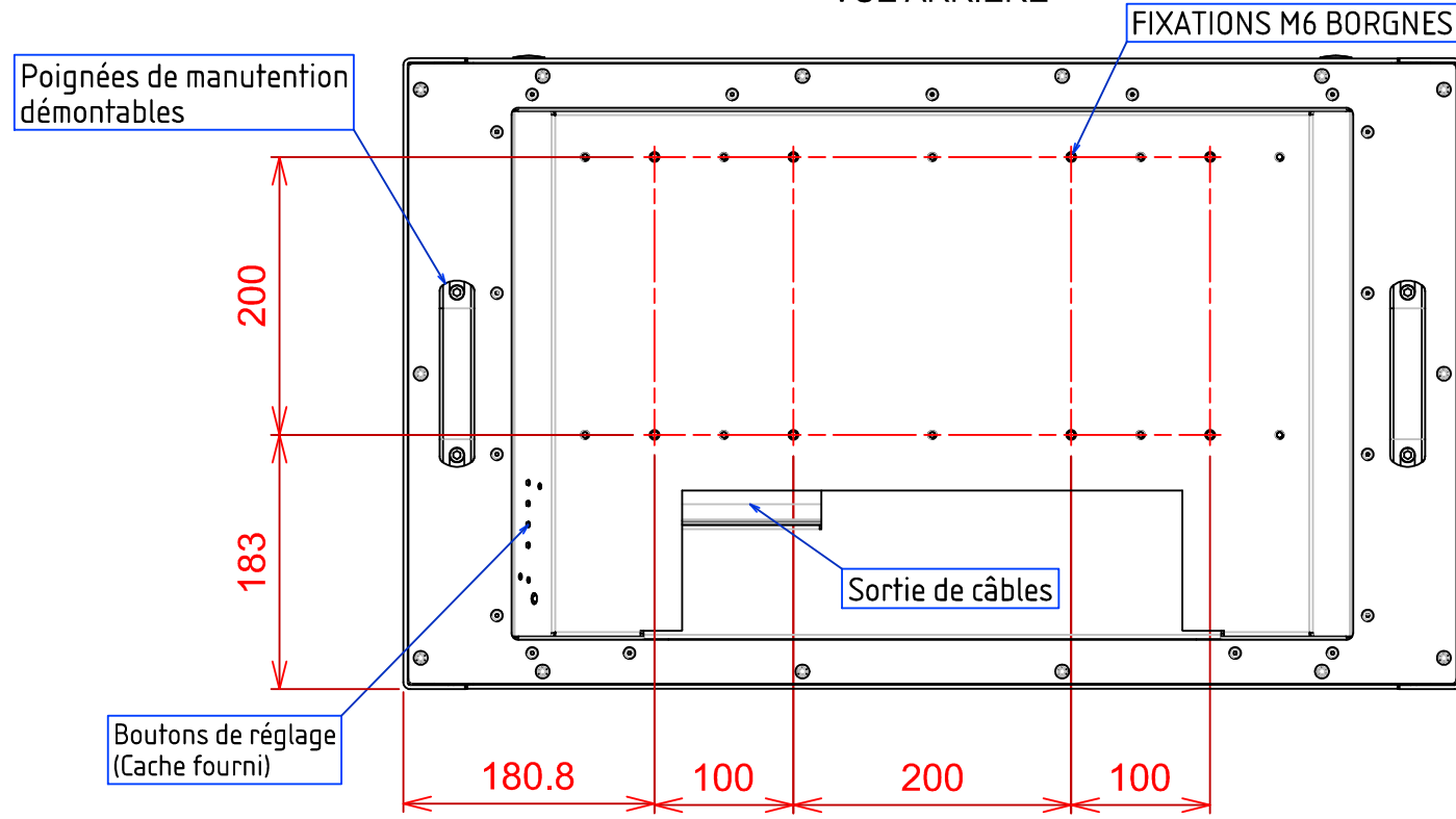
VUE ARRIERE
